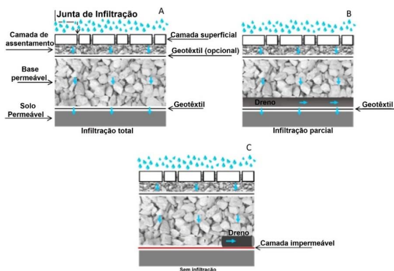
Figura 15. Capacidade de infiltração do pavimento permeável.
