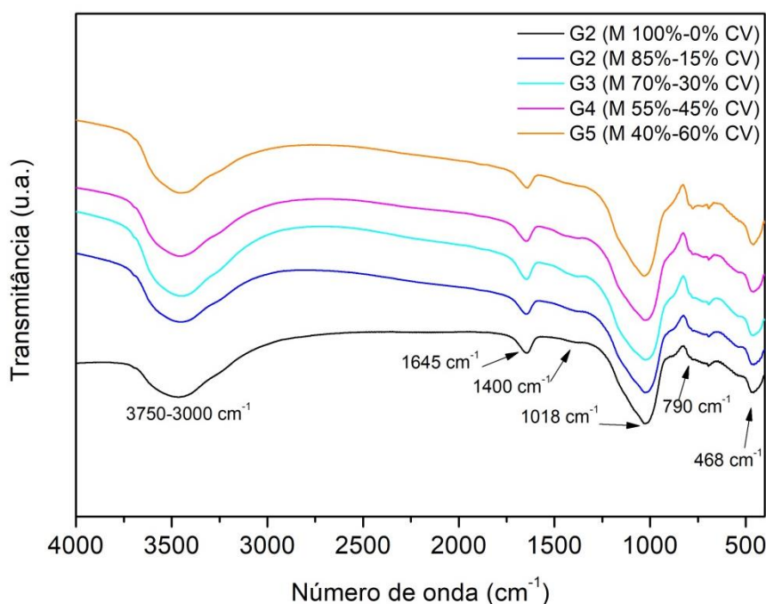
Figura 26. Espectros no infravermelho dos produtos geopoliméricos com diferentes proporções dos precursores.
