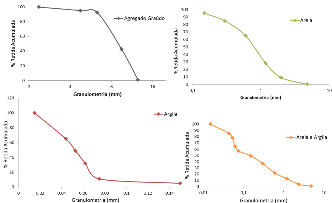
Figura 36. Curva granulométrica das amostras.
