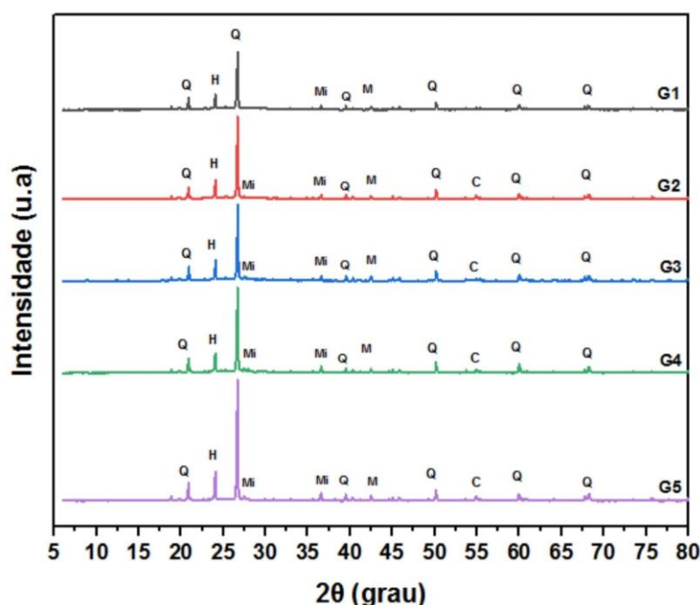
Figura 25. Difrátogramas dos geopolímeros onde Q, H e M correspondem a Quartzo, Hematita e Muscovita.
