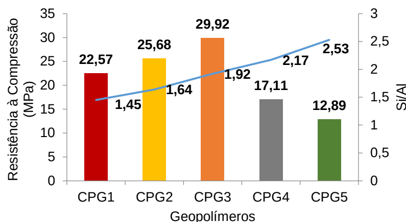
Figura 43. Resultado do ensaio de resistência à compressão.
