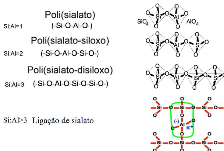
Figura 5: Classificação dos diferentes tipos de geopolímeros.
