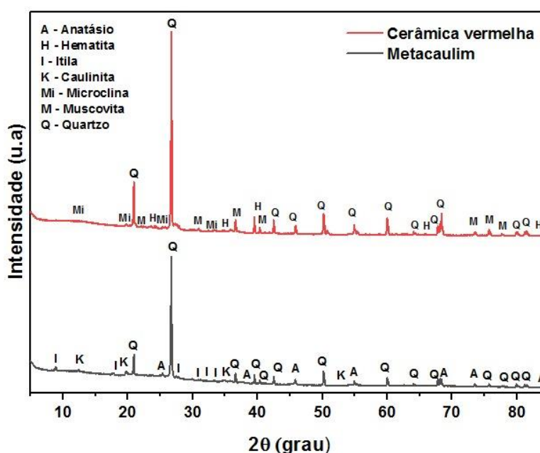
Figura 35. Difratograma de raios-X dos precursores.
